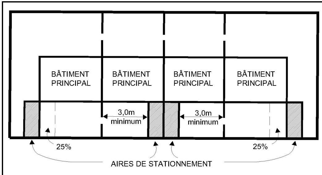
CROQUIS 35 : LOCALISATION DES AIRES DE STATIONNEMENT POUR LES HABITATIONS EN RANGÉE
