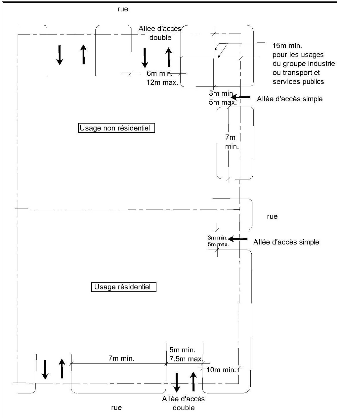
CROQUIS 33 : DISTANCE ET LARGEUR DES ALLÉES D'ACCÈS À LA PROPRIÉTÉ SIMPLE ET DOUBLE
