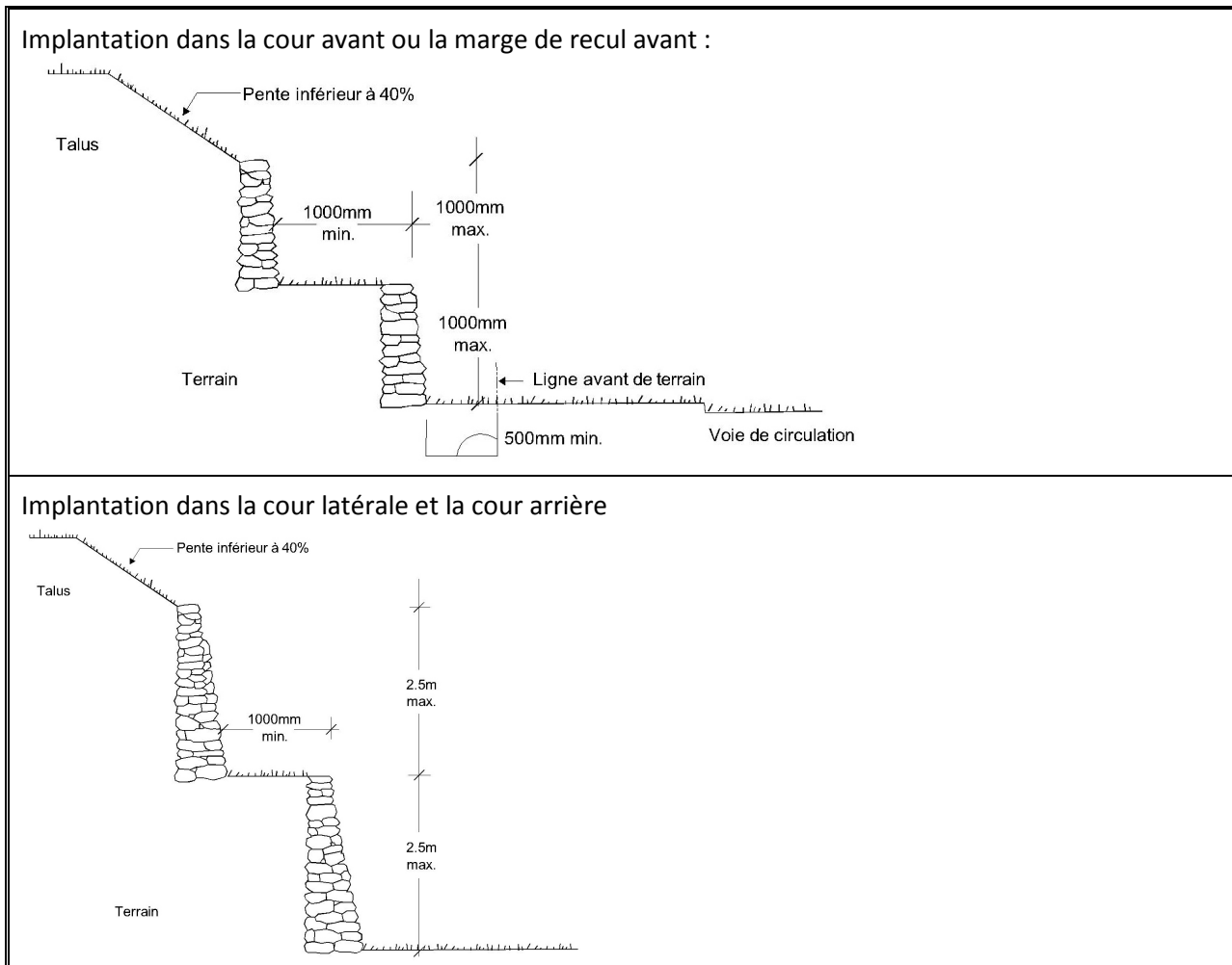
CROQUIS 32 : IMPLANTATION D'UN MUR DE SOUTÈNEMENT DANS LES COURS ET MARGES DE REcul
