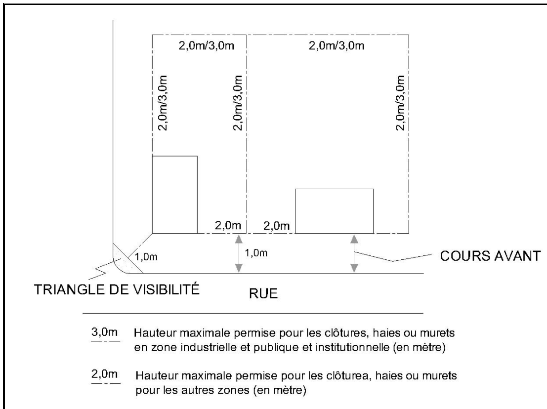
CROQUIS 31 : IMPLANTATION D'UNE CLÔTURE, D'UN MUR ET D'UNE HAIE
