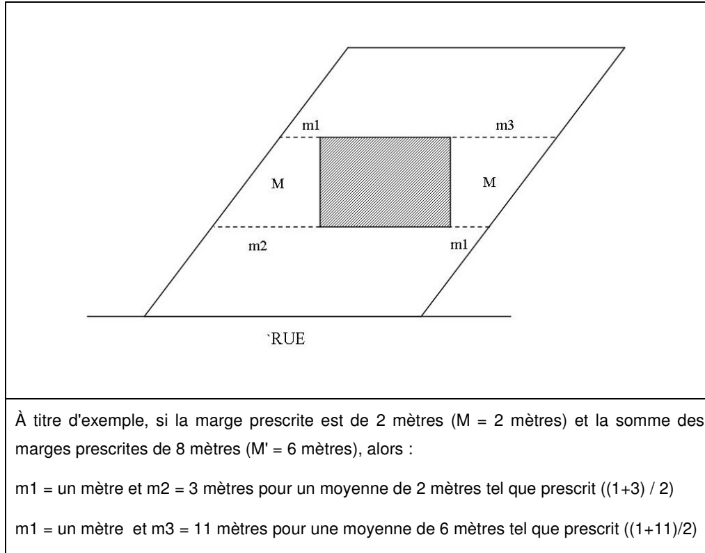
CROQUIS 25 : MARGE DE REcul LATÉRALE DANS LE CAS D'UN TERRAIN PARALLÉLOGRAMME
