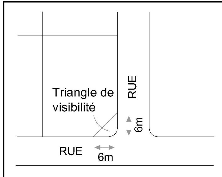
CROQUIS 30 : TRIANGLE DE VISIBILITÉ
